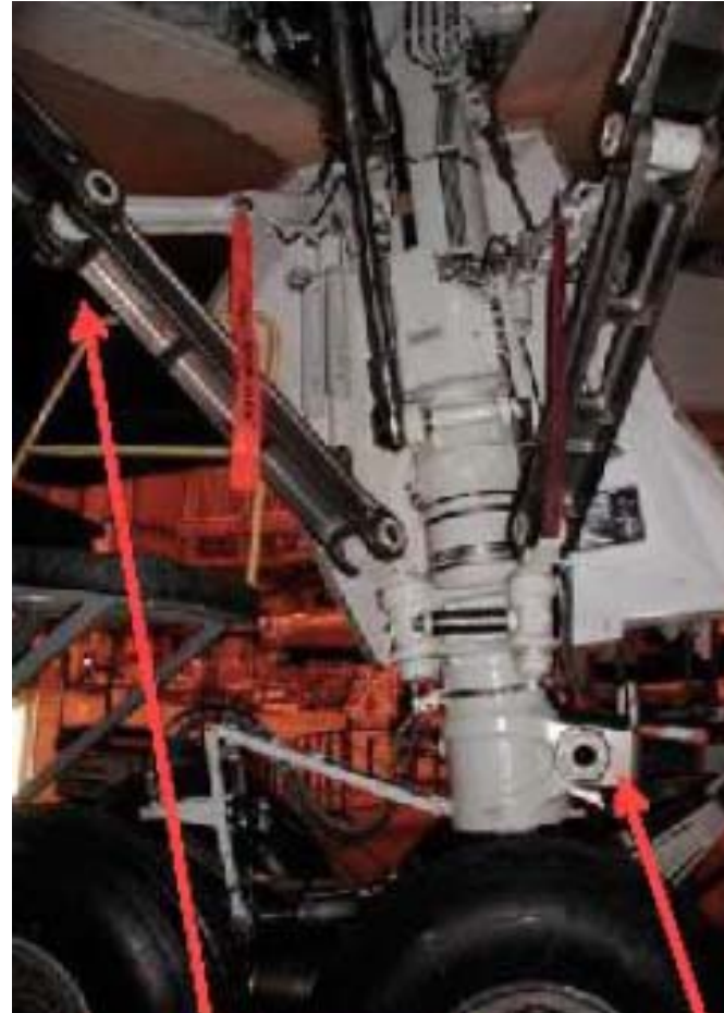
Элементы основной стойки шасси
